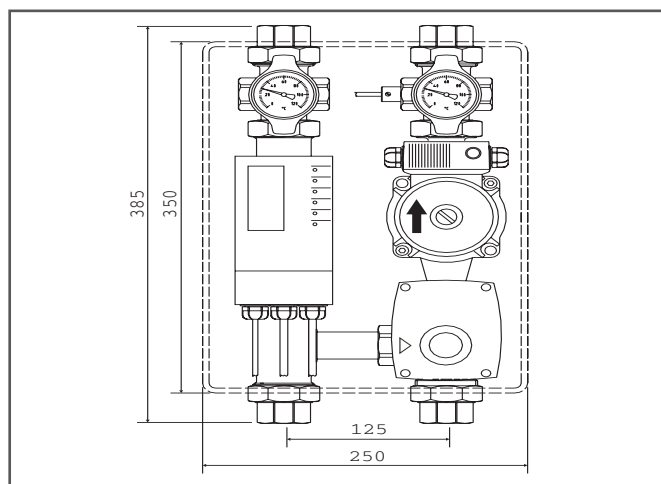
Fig. 7-8 Unitatea de reglare a temperaturii REHAU TRS-20
