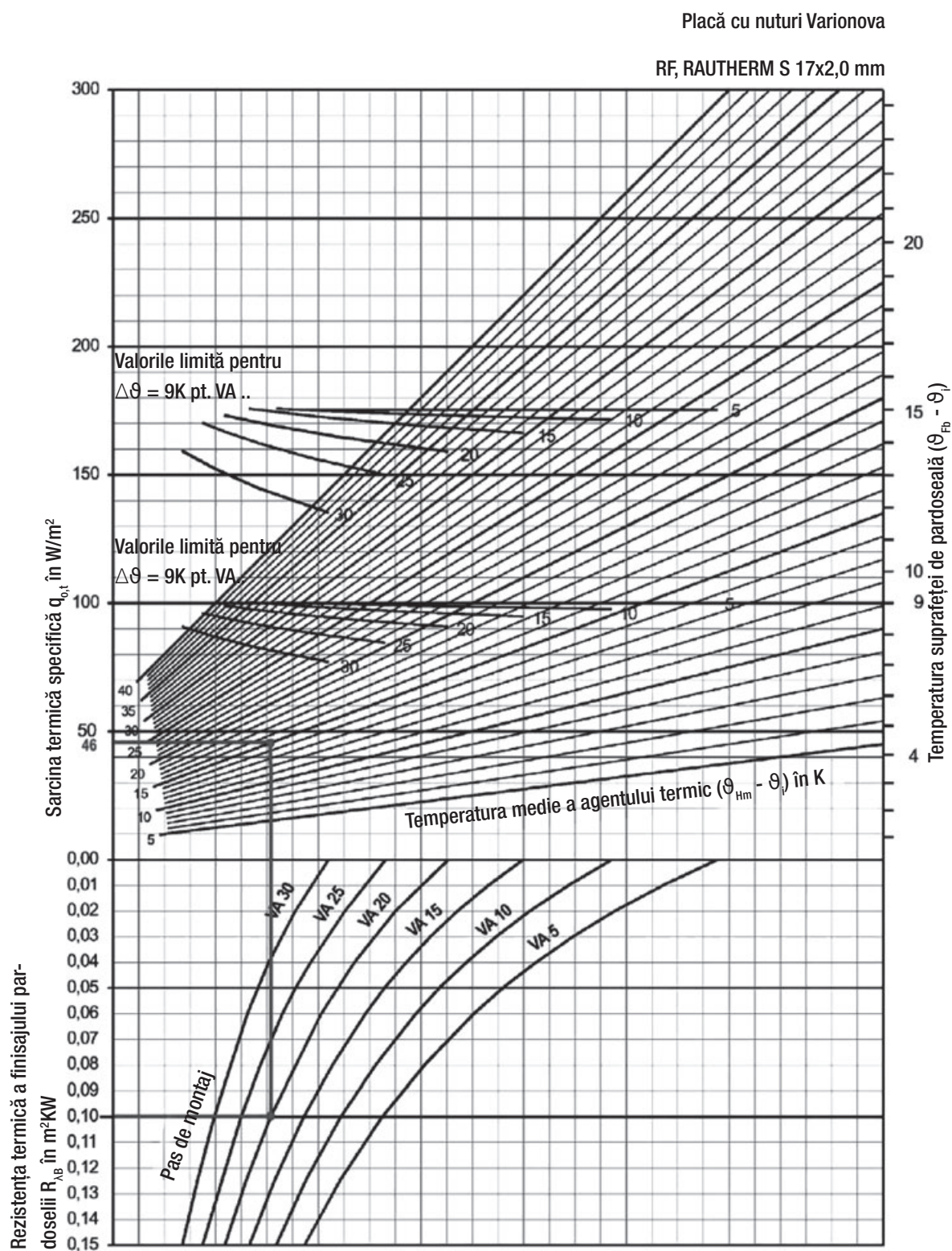
Fig. 10-2 Diagrama de dimensionare termică
