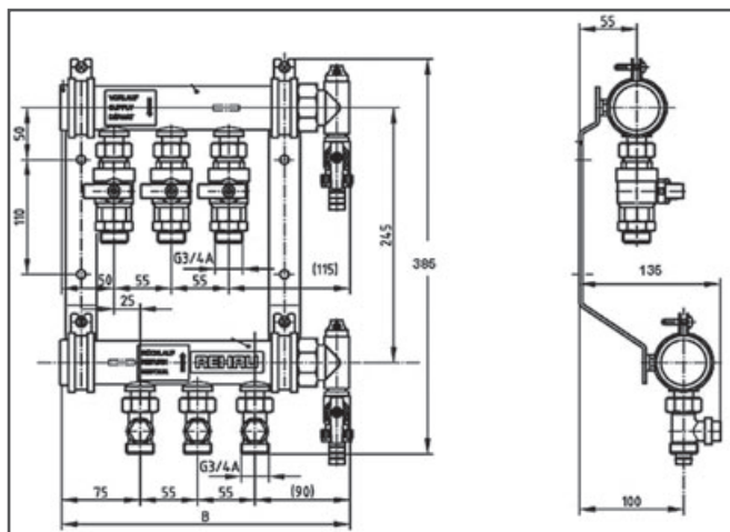
Fig. 9-40 Dimensiuni
