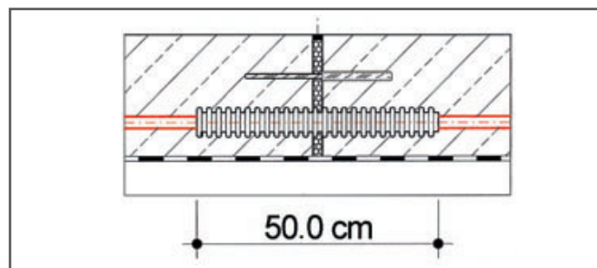
Fig. 9-11 Rost de dilatare îmbinat cu cep Țeavă de protecție REHAU
