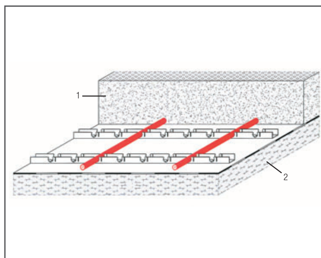
Fig. 9-9 Placă de pardoseală armată cu ace; construcție standard – țevele de încălzire montate pe șine cu cleme
