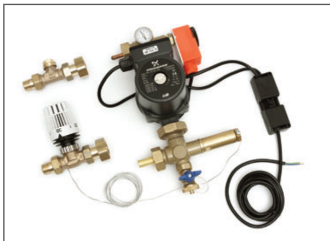
Fig. 7-4 Kit REHAU pentru reglarea temperaturii agentului termic
