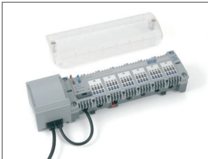
Fig. 7-15 Distribuitor REHAU de reglare EIB
