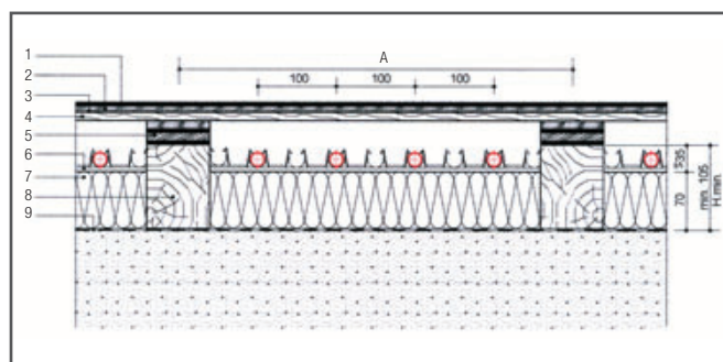
Fig. 9-20 Structura sistemului de încălzire prin pardoseală
