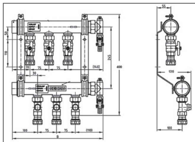
Fig. 9-36 Dimensiuni
