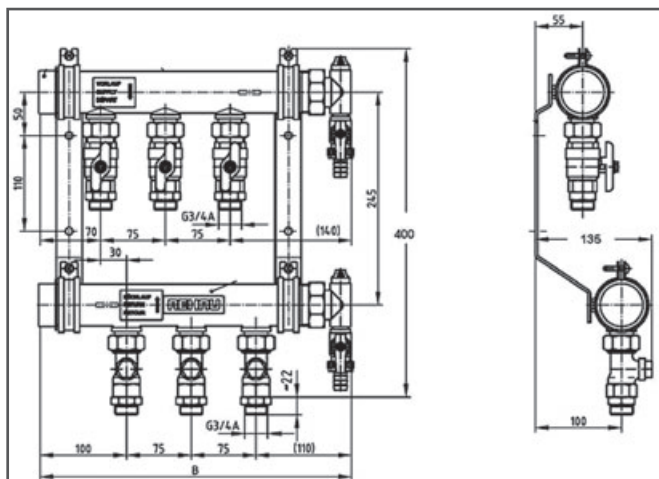
Fig. 9-38 Dimensiuni
