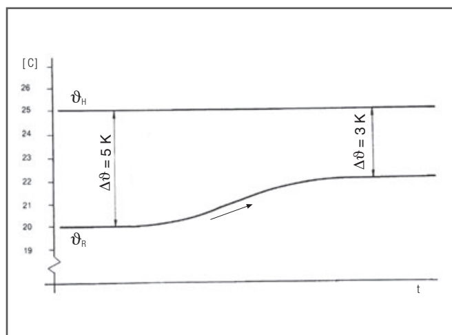
Fig. 7-1 Efectul de autoreglaj
