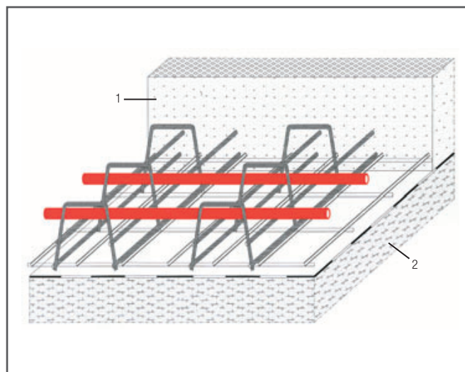
Fig. 9-7 Placă de pardoseală armată cu pat de oțel; construcție standard – țevele de încălzire montate pe patul inferior de armătură
