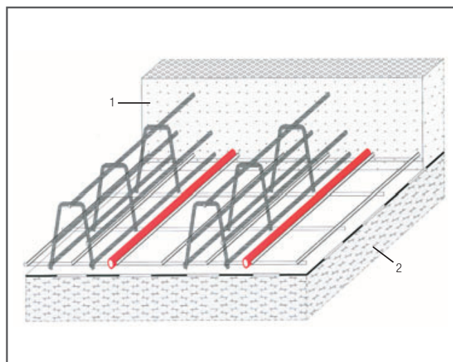
Fig. 9-8 Placă de pardoseală armată cu pat de oțel; construcție standard – țevele de încălzire montate central în placă
