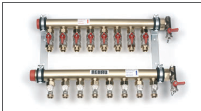
Fig. 9-35 Distribuitor industrial REHAU 1 1/4" IVK
