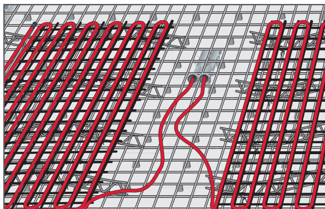
Fig. 8-29 Pasul 3: Montajul modulelor REHAU BKT
