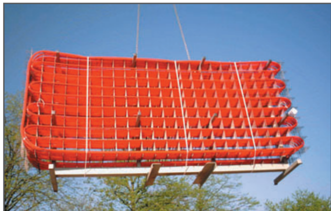
Fig. 8-26 Suport de transport REHAU-BKT
