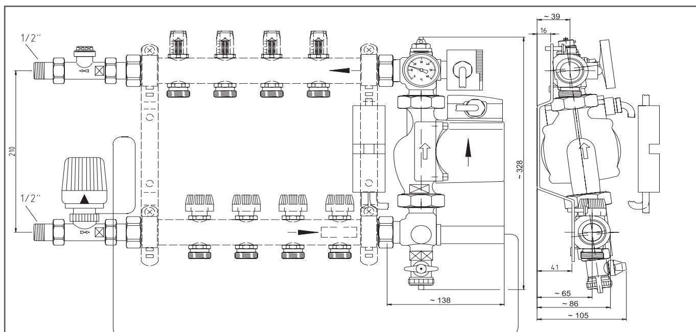
Fig. 7-5 Kitul de reglare a temperaturii agentului termic cu HKV-D
