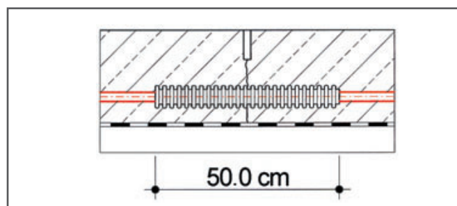
Fig. 9-12 Rost aparent, rost de zi Țeavă de protecție REHAU
