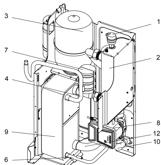
4/6 kW unitate cu încălzitor de a rezervă (opțional)
