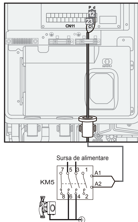
Pompă P_d conductă ACM:
