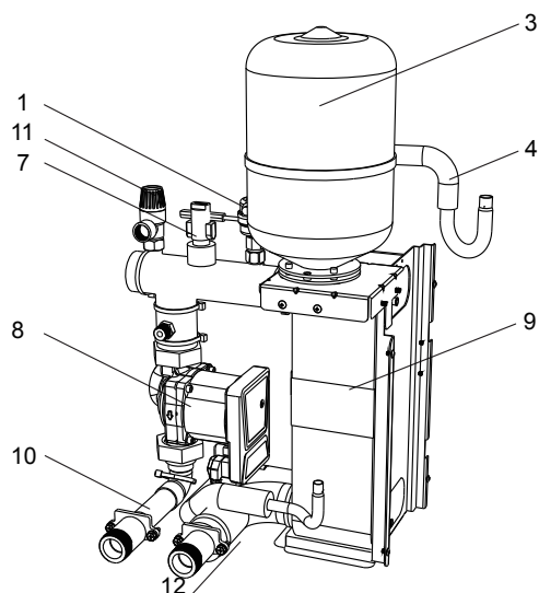
4/6 kW unitate fără încălzitor de a rezervă
