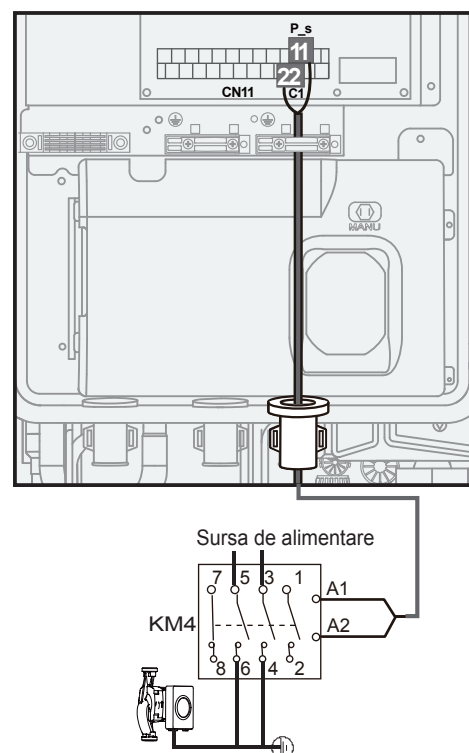
Pompă P_s energie solară:
