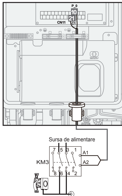
Pompă P_o de circulație suplimentară:
