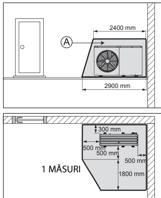
Amplasarea unității exterioare într-un colț, spre stânga
