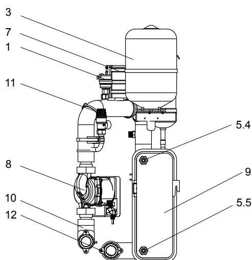
4/6 kW unitate fără încălzitor de a rezervă
