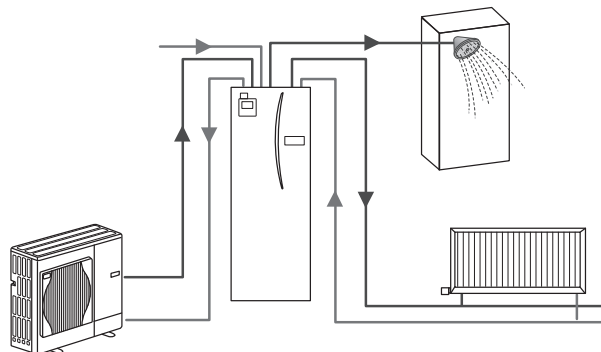
Schéma de l'ensemble Ecodan hydrobox duo
