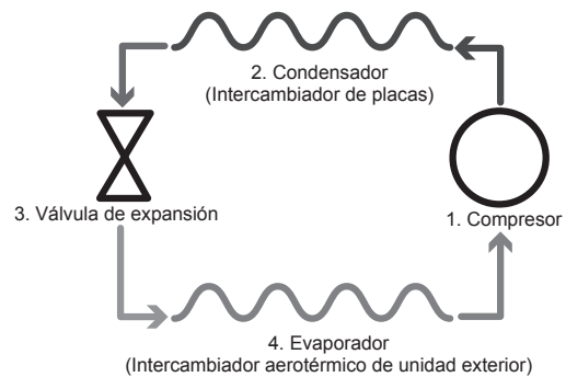
Esquema del sistema duo compacto
