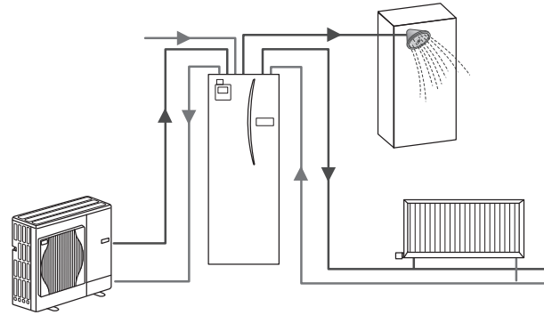
Darstellung der Wärmepumpenanlage mit Speichermodul
