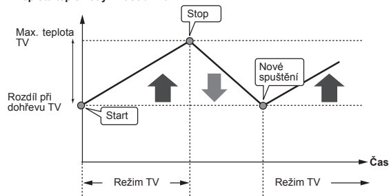
Teplota teplé vody v zásobníku TV
