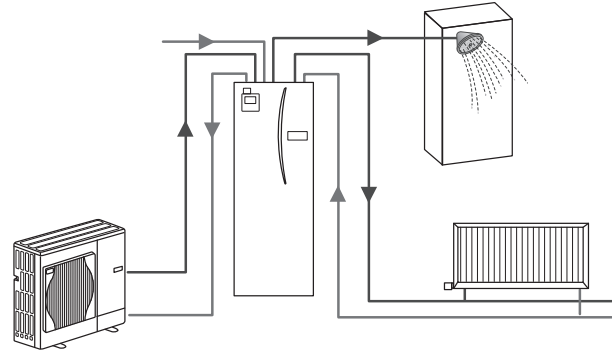
Esquema do sistema de cilindro compacto
