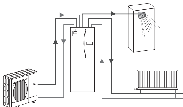
Schema di impianto monoblocco con hydrotank
