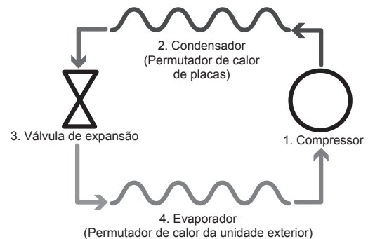
Esquema do sistema de cilindro compacto
