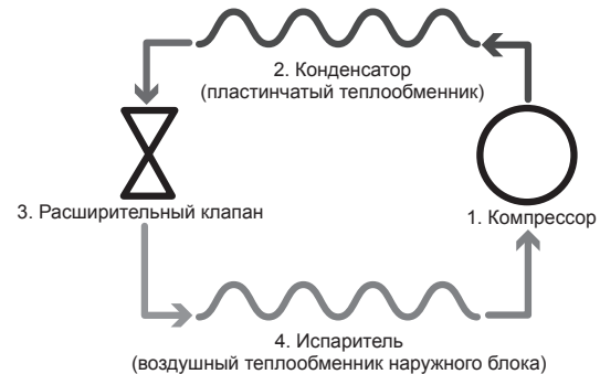
Принципиальная схема системы нагрева воды
