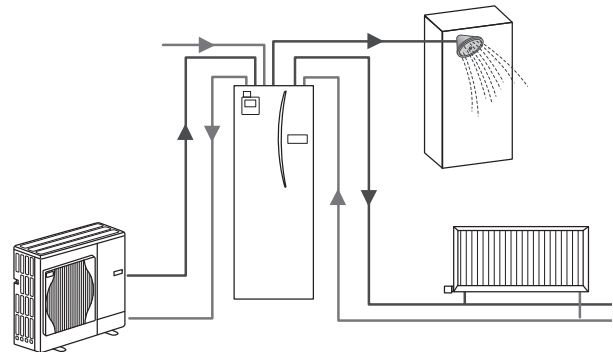
Oversikt over ferdigmontert sylindersystem
