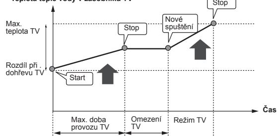
Teplota teplé vody v zásobníku TV
