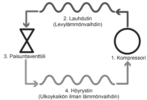
Pakettivaraajajärjestelmän kaavioesitys
