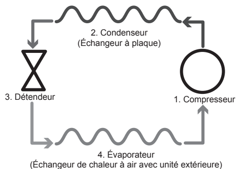
Schéma de l'ensemble Ecodan hydrobox duo
