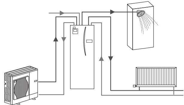
Schematische voorstelling monobloc-systeem
